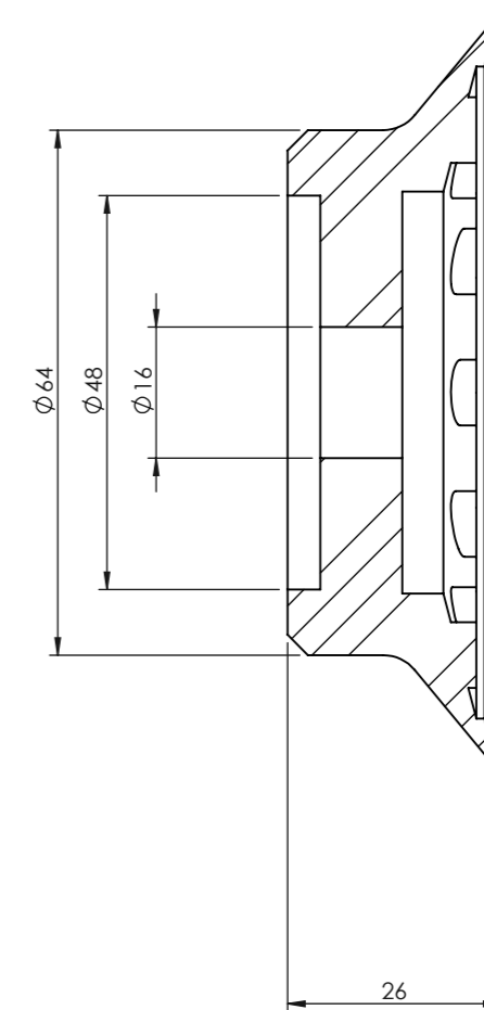
SEZIONE A-A
